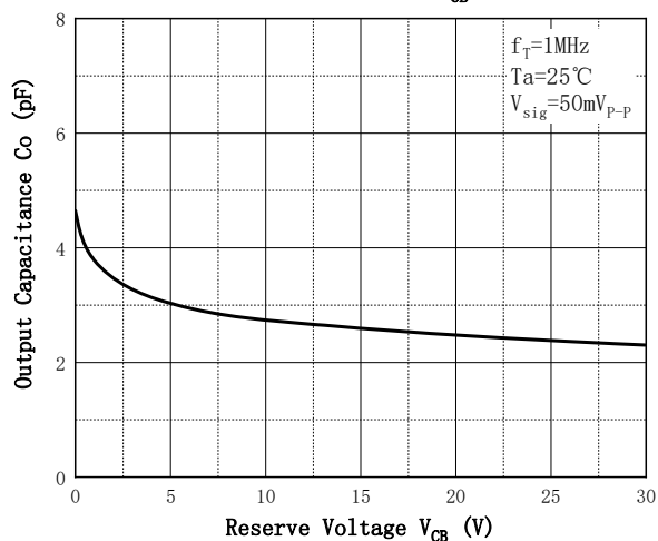
Fig.5 - C_o — V_{CB}
